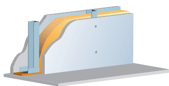
pojedyncza konstrukcja nośna – pojedyncze oplytowanie
