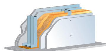
podwójna konstrukcja nośna – podwójne oplytowanie
