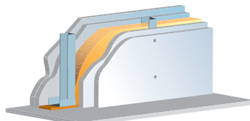
pojedyncza konstrukcja nośna – podwójne oplytowanie
